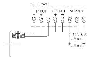
Misure di velocità con captatore alimentato (12V c.c.) Powered proximity (12V d.c.) speed measurements
