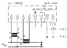
Wattmetro - Varmetro - Cosfimetra per linea monofase Wattmeter - Varmeter - Power - Factor meter for single wires
